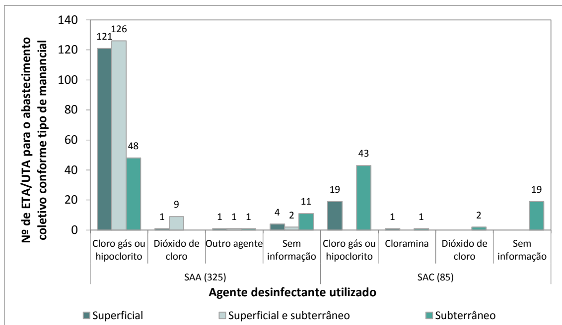
Figura 5.37 - Quantidade de ETA/UTA por tecnologia de desinfecção, tipo de sistema e característica do manancial
