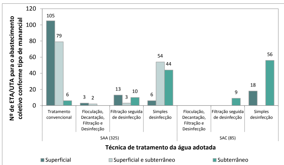
Figura 5.35 – Quantidade de ETA/UTA por tecnologia de tratamento, tipo de sistema e característica do manancial
