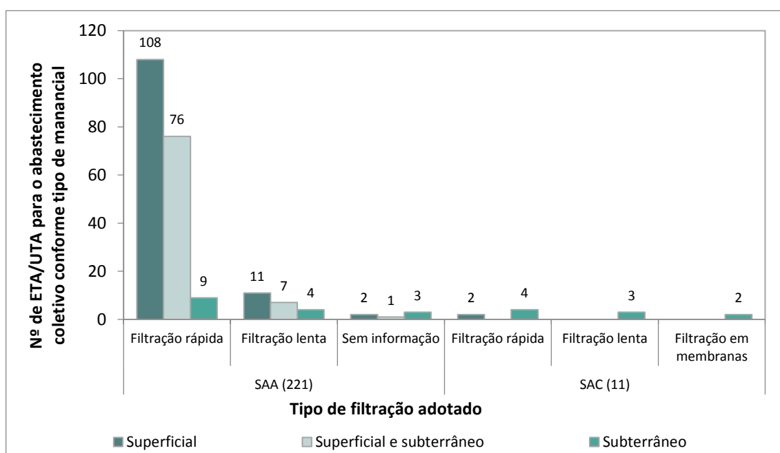
Figura 5.36 - Quantidade de ETA/UTA por tecnologia filtração, tipo de sistema e característica do manancial
