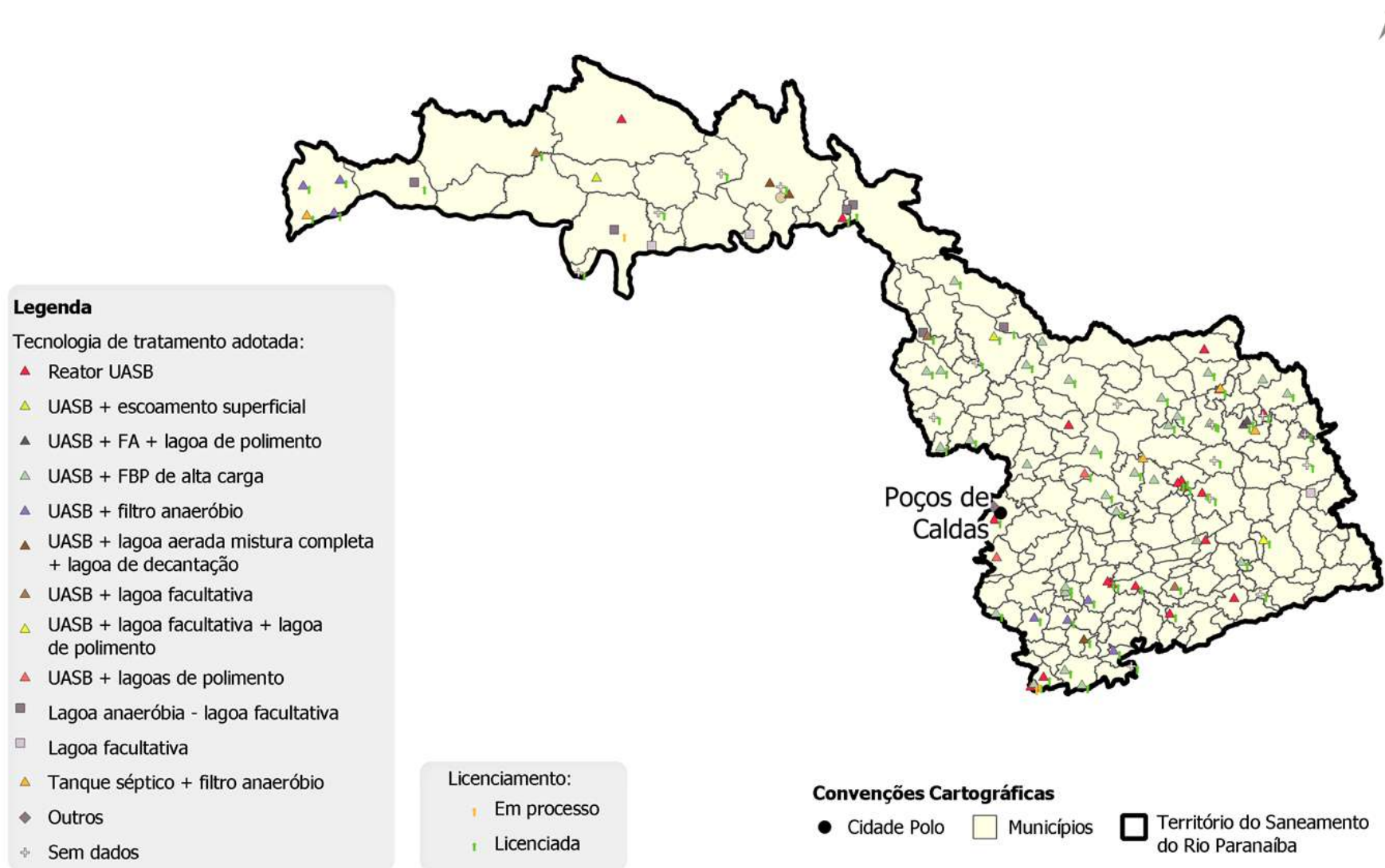
Figura 5.84 –Tecnologias de tratamento adotadas nas ETE do TS-5 e situação do licenciamento
